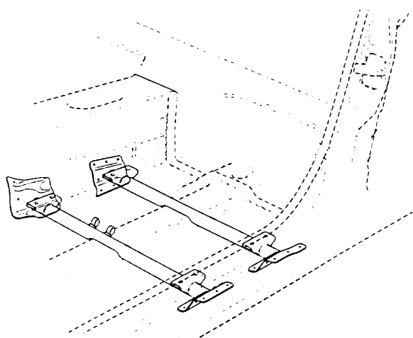
Рис. 2 Крепление сиденья
